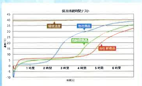
試験条件: 家庭用冷凍庫(-20℃設定)の12時間以上冷却させた保冷剤の冷却面の保冷持続時間を環境温度約40℃で測定を行った。
